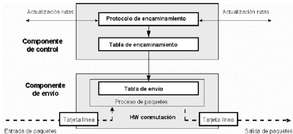
Ilustración 6. Fuente: http://exa.unne.edu.ar/informatica/SO/MPLS.PDF
