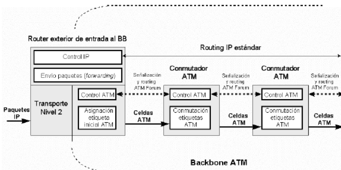
Ilustración 5. Fuente: http://exa.unne.edu.ar/informatica/SO/MPLS.PDF
