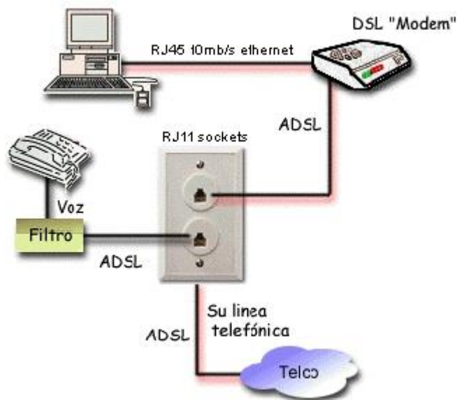
Ilustración 2. Fuente: https://sites.google.com/site/historiayconceptosdelinternet/internet/tipos-de-conexion/adsl
