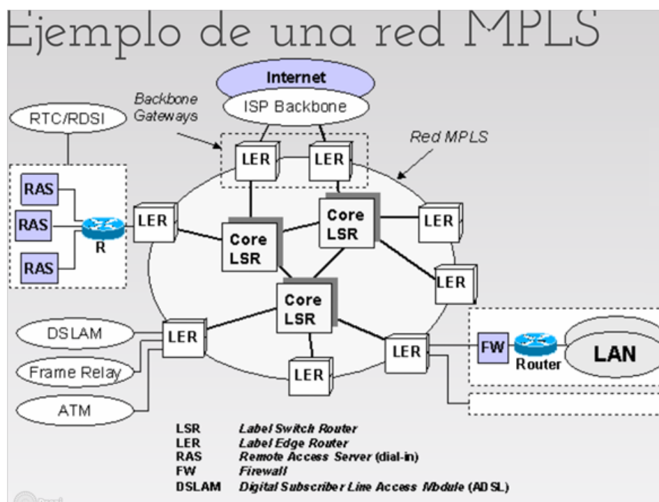
Ilustración 9. Fuente: http://calidaddeservicioteleprocesos.blogspot.com.ar/2016_04_01_archive.html
