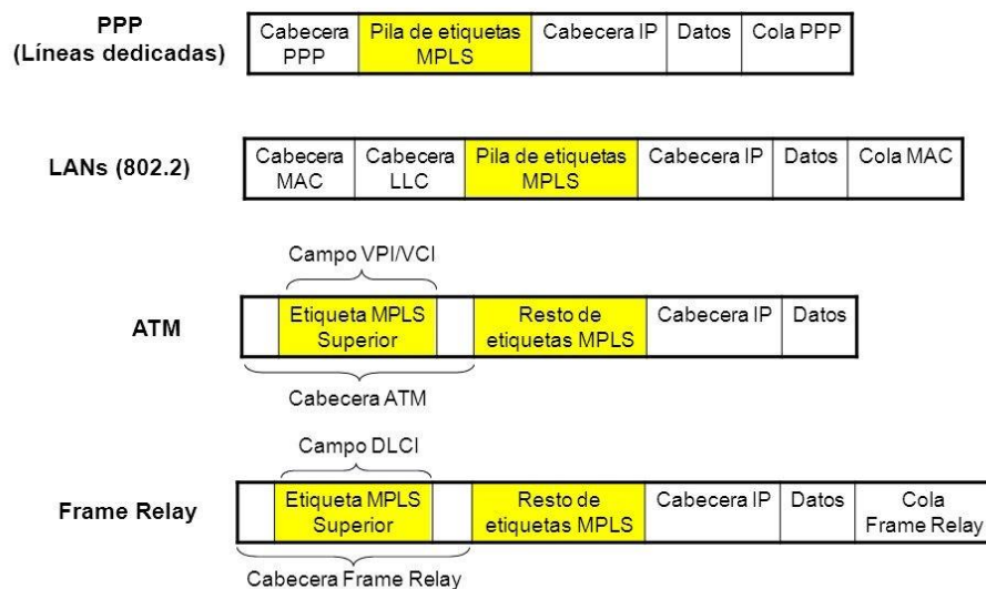
Ilustración 12. Fuente: http://slideplayer.es/slide/10897165/
