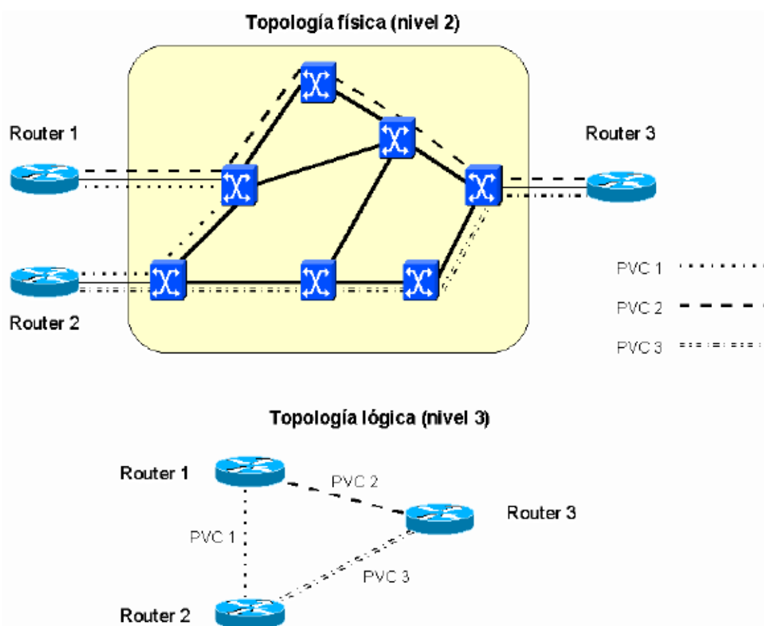
Ilustración 4. Fuente: http://exa.unne.edu.ar/informatica/SO/MPLS.PDF
