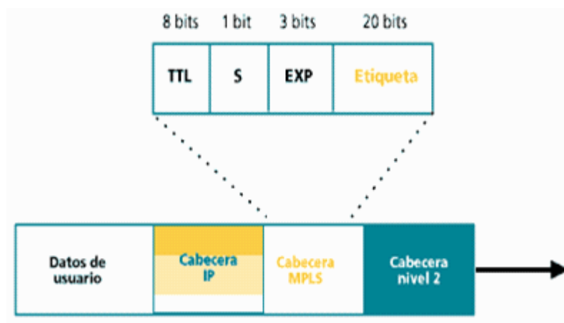
Ilustración 10. Fuente: http://www.monografias.com/trabajos29/informacion-mpls/informacion-mpls.shtml
